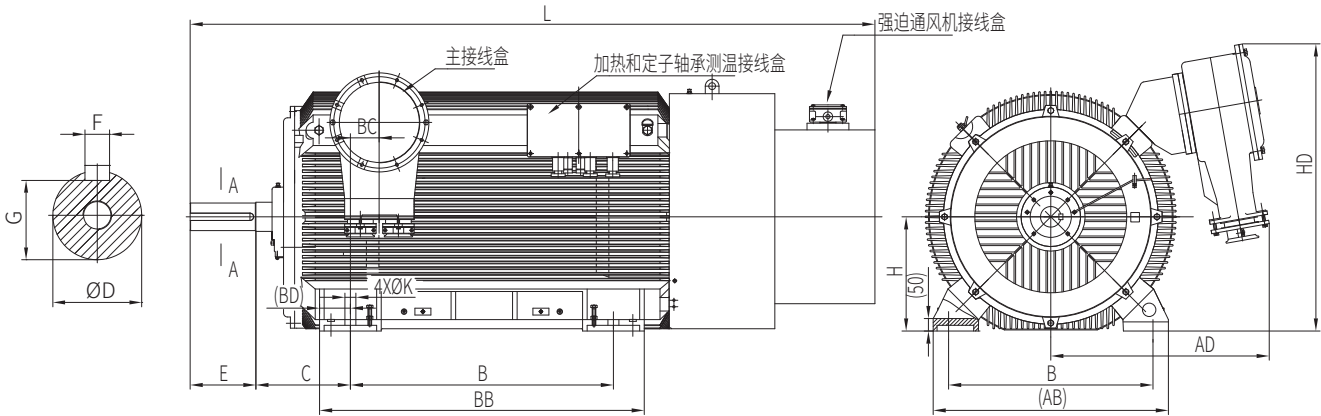
YBBP-400~560 电动机安装方式及外型尺寸
